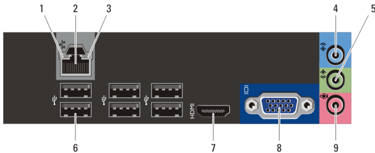
Ilustración 3. Vista del panel posterior de la minitorre y del equipo de escritorio
