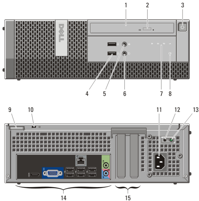
Ilustración 4. Vista frontal y posterior del factor de forma pequeño
