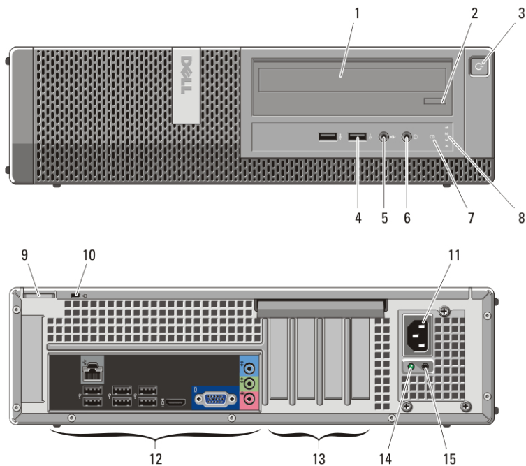
Ilustración 2. Vista frontas y posterior del equipo de escritorio
